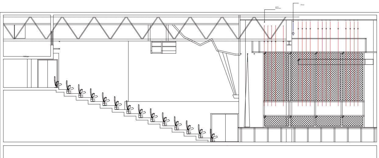
Coupe longitudinale
