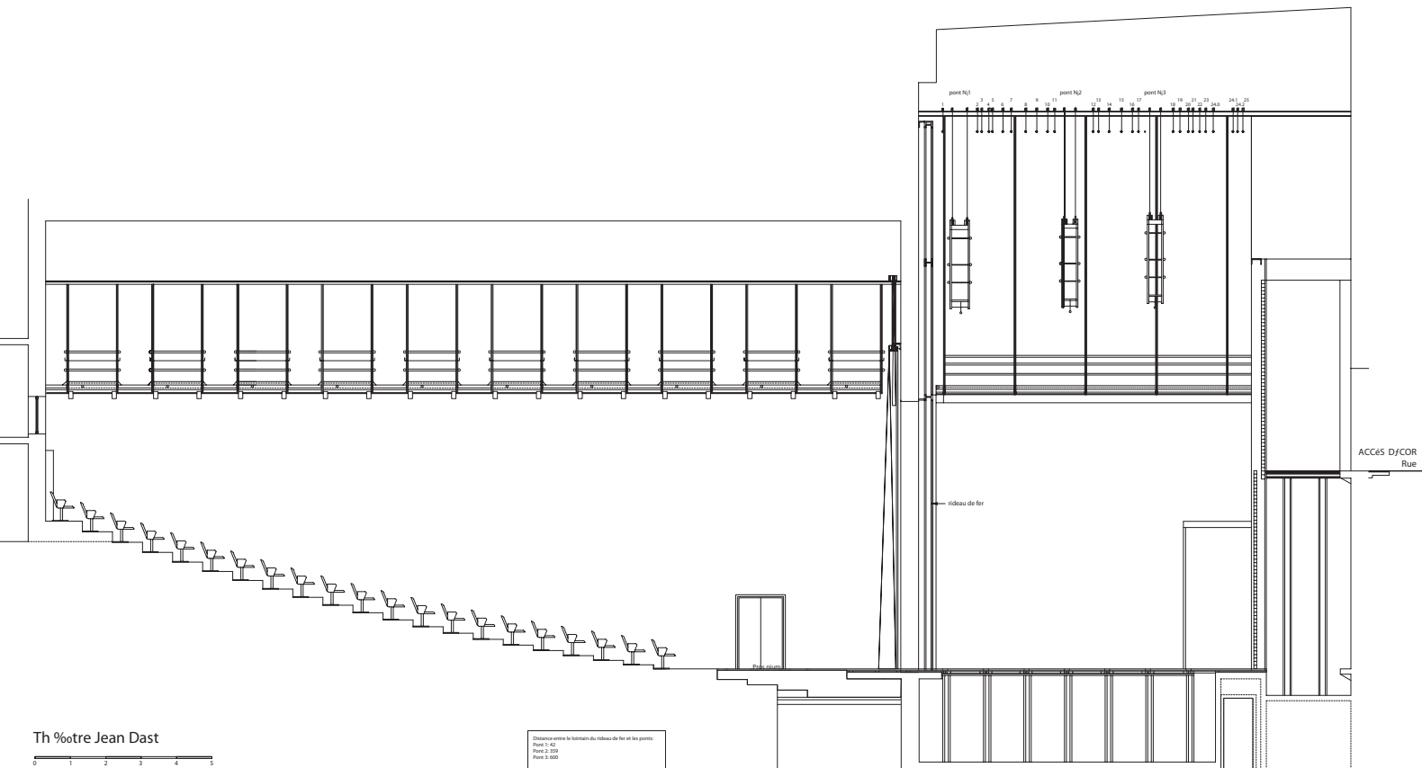
Coupe longitudinale
